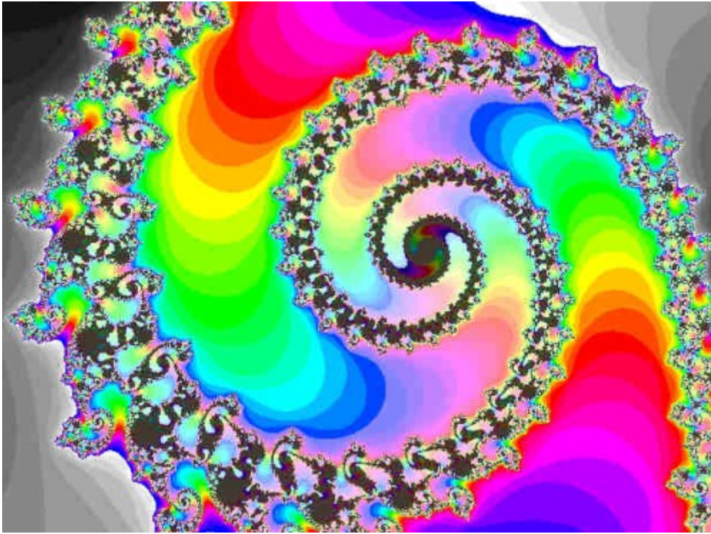
FRACTALE de Julia
